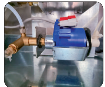
Pompa elettromagnetica (di serie)
